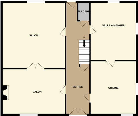
REZ-DE-CHAUSSEE
